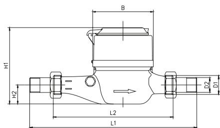
Dimensiones MTKD-S
